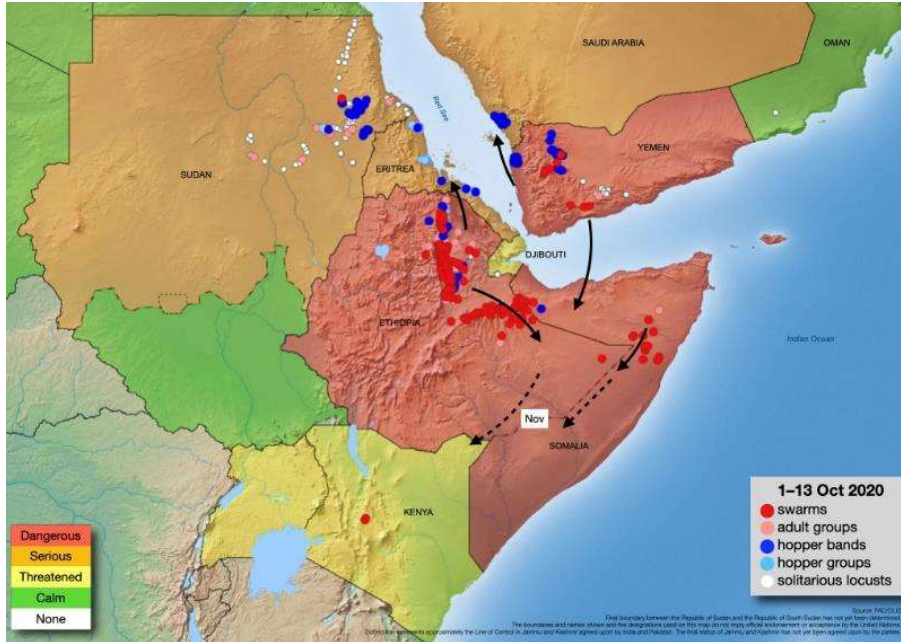
حالة الجراد الصحراوي تحديث 14 أكتوبر 2020
